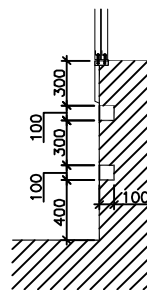
DETALLE PATES DE FOSO
