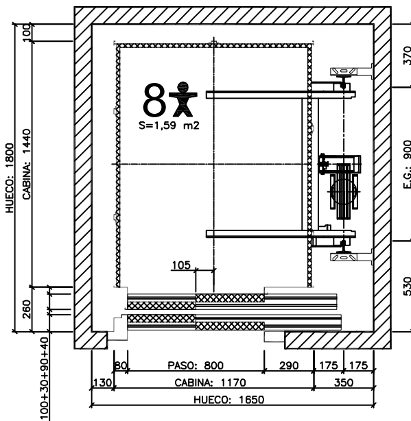
PLANTA DE PISOS
