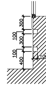
DETALLE PATES DE FOSO
